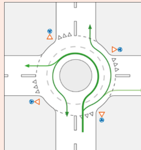
Abbildung mehrspuriger Kreisel.
